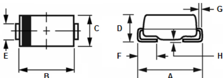
DO-214AA / SMB
